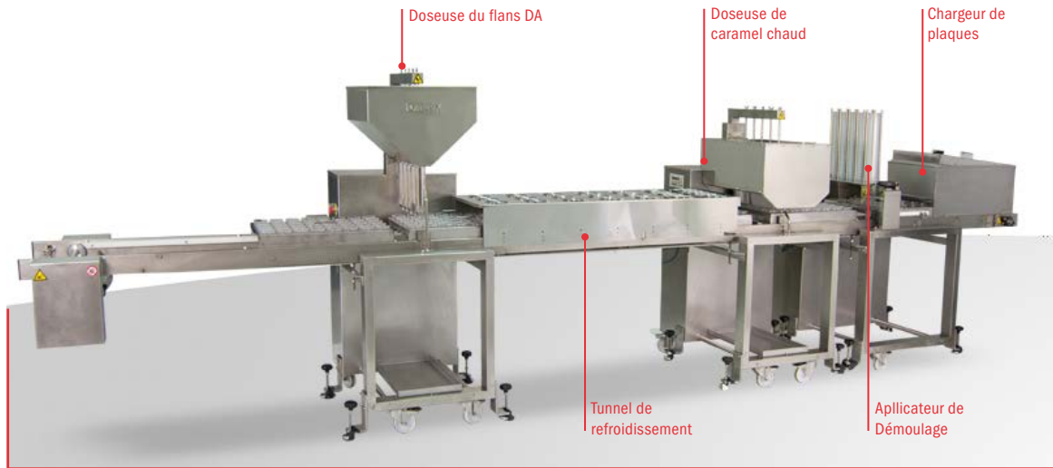
Ligne de production modulaire pour flan
