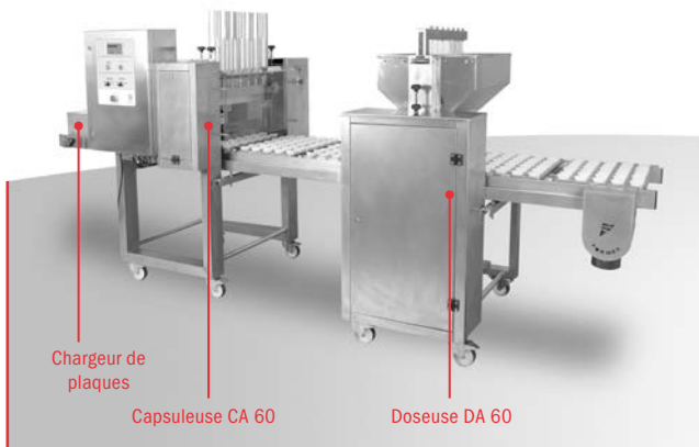
Ligne de production modulaire pour madeleines
