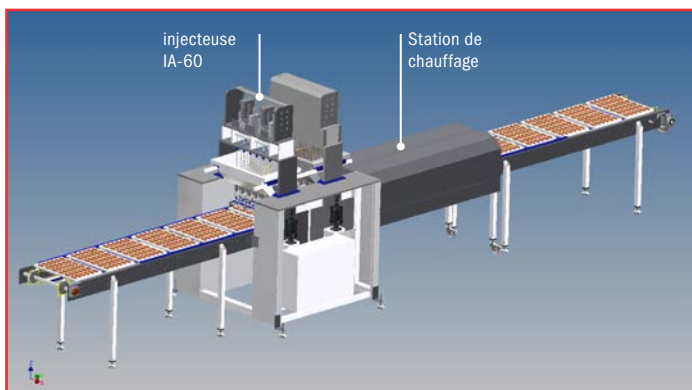
Ligne modulaire pour l'injection de croissants avec double trémie
